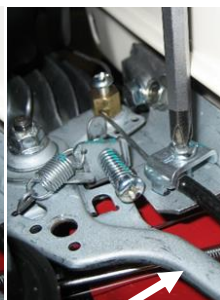
4 ANEXAR A TAMPA DO ACELERADOR
